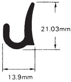
J19 0.089 kg/ft 0.29 kg/m
