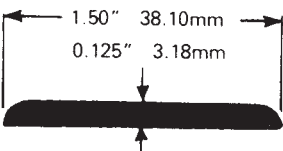
DR3 0.101 kg/ft 0.33 kg/m
