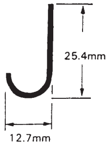
J4 0.050 kg/ft 0.17 kg/m
