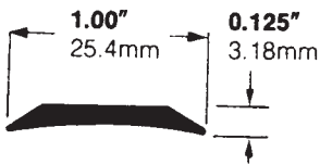
DB1 0.049 kg/ft 0.16 kg/m
