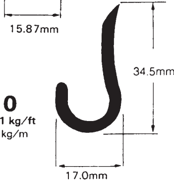
CC5 0.110 kg/ft 0.36 kg/m
