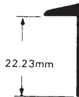
EC1 0.09 kg/ft 0.30 kg/m
