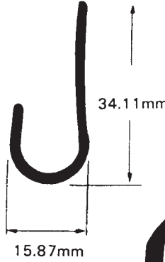
J6 0.091 kg/ft 0.30 kg/m
