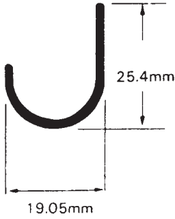
J5 0.063 kg/ft 0.21 kg/m
